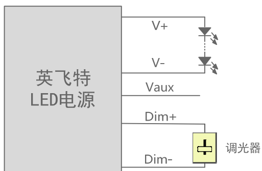
示意图 2：负逻辑
